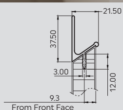
Shutter Handle 1936 Mitre Cut
